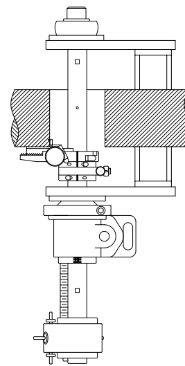
Grooving
